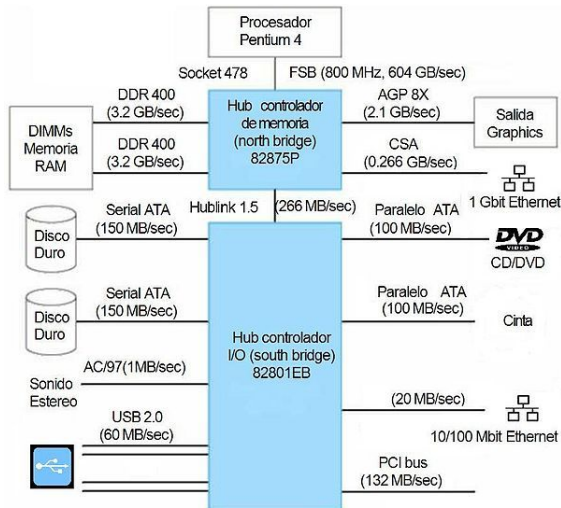
Chipset 875 de Intel, usado con procesadores Pentium 4 en encapsulado de pines.
