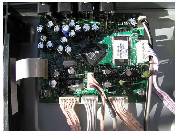
Circuito impreso de un DVD Philips, se puede apreciar el chipset MT1389 del fabricante MediaTek y los pocos componentes auxiliares como el controlador de servos (abajo a la izquierda) y la memoria flash (derecha).
